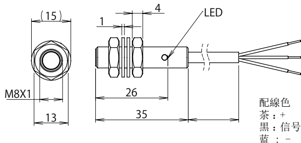
连线图 C012/P. 102
