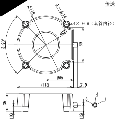
传送头
