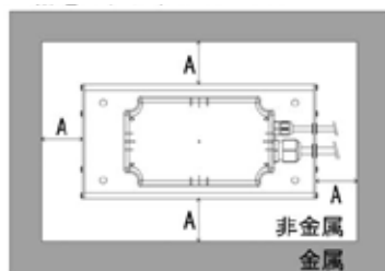
■標準仕様給電ヘッド RCS600-AH
