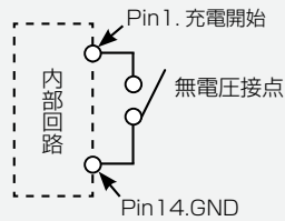
A 接点仕様
