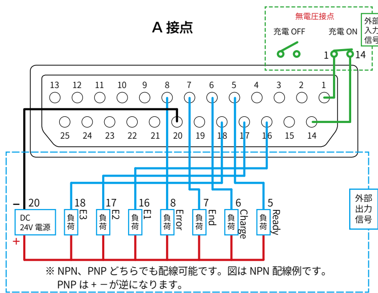
コネクタ（ケーブル配線側）の嵌合面
