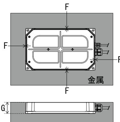
■長距離仕様給電ヘッド／RCS600-AH-L
