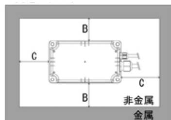
■標準仕様受電ヘッド RCS600-CH
