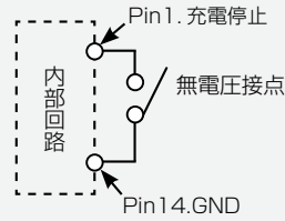
B 接点仕様
