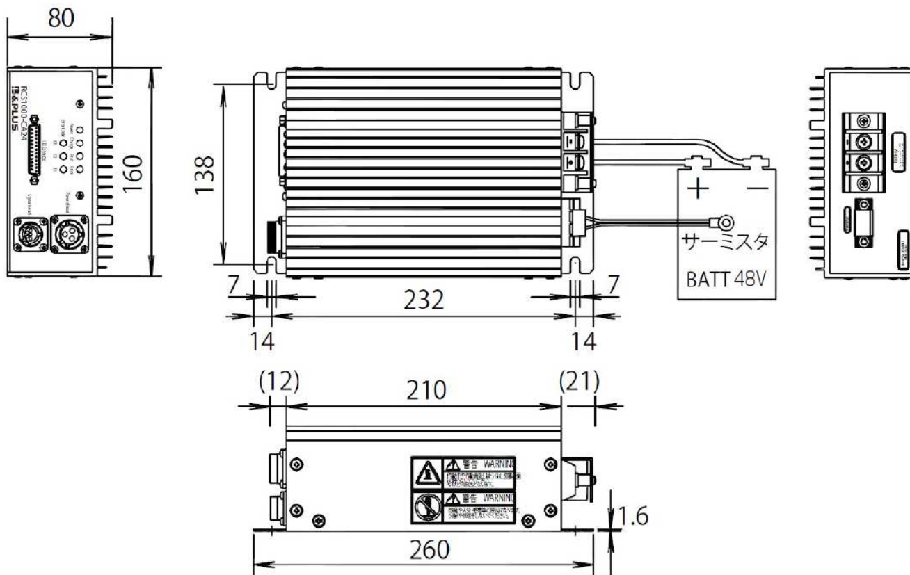
外形寸法図
