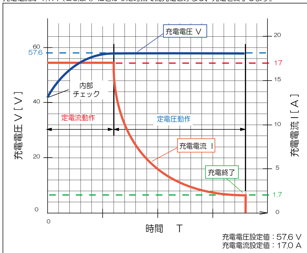
[ 充電制御グラフの例 ]
