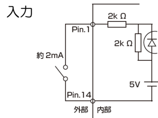
入力信号回路図 Fig.34
