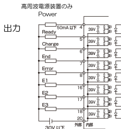
出力信号回路図 Fig.35
