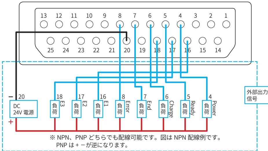
コネクタ（ケーブル配線側）の嵌合面
